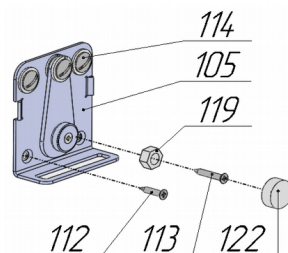
Рис.10.1 Закрепление при установке механизма на ЛЕВОМ щите короба
